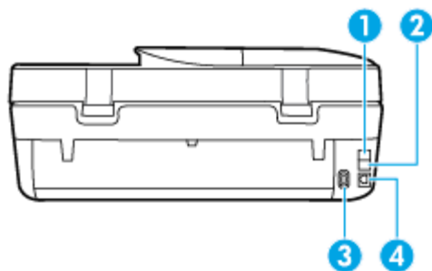
Rysunek 2-2 Widok z tyłu urządzenia HP OfficeJet 4650 All-in-One series
