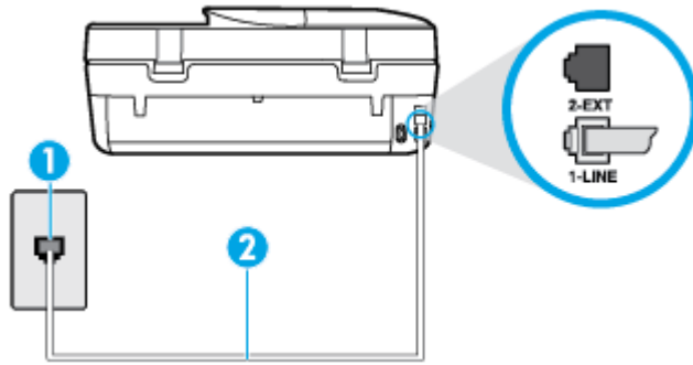
Figura B-5 Vista posterior do dispositivo
