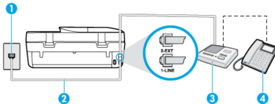
Figura B-11 Vista posterior do dispositivo
