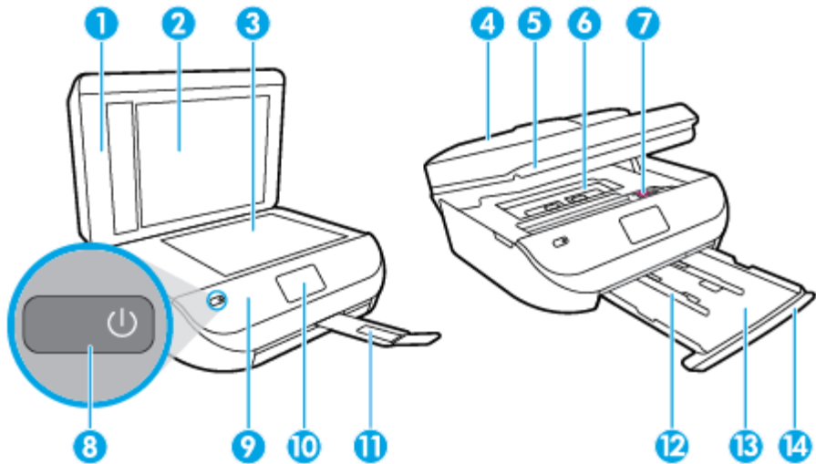
Рисунок 2-1 Вид HP OfficeJet 4650 All-in-One series спереди и сверху
