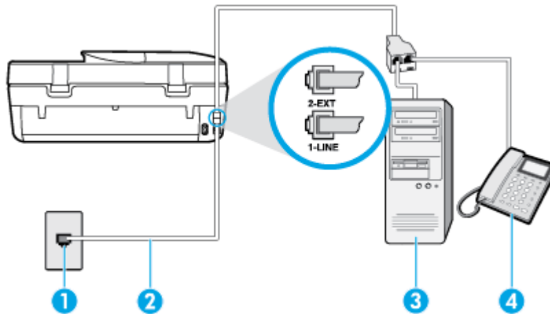
圖示 B-16 印表機的背視圖
