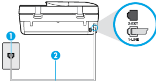
圖示 9-1 印表機的背視圖
