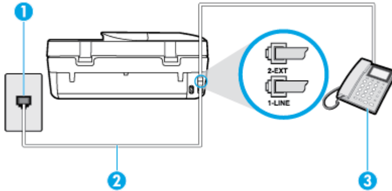
圖示 B-4 印表機的背面檢視
