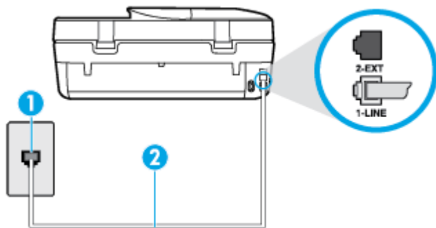
圖示 B-5 印表機的背視圖
