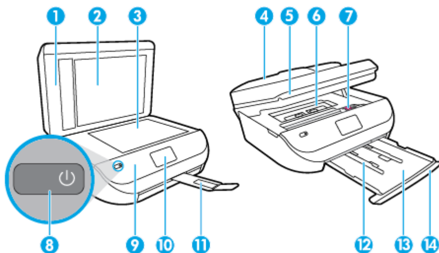
圖示 2-1 HP OfficeJet 4650 All-in-One series 的前視圖與俯視圖
