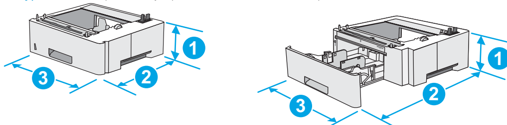
Фигура 1-3 Размери за 1 х устройство за подаване на хартия за 550 листа
