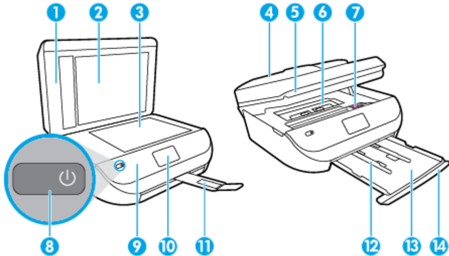
図 2-1 HP DeskJet Ink Advantage 4670 All-in-One series の正面および上面図
