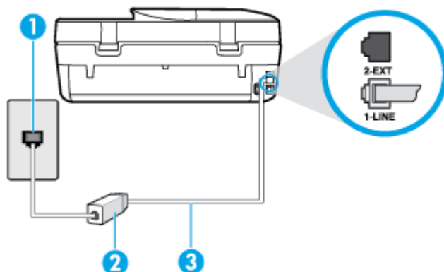
図 B-2 プリンターの背面図
