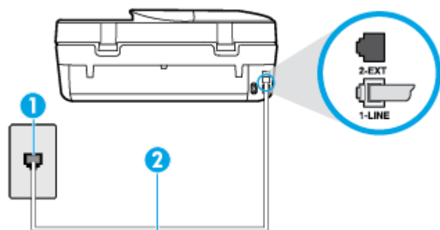
図 9-1 プリンターの背面図
