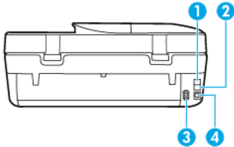
그림 2-2 HP DeskJet Ink Advantage 4670 All-in-One series 뒷면
