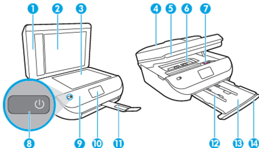
图 2-1 HP Deskjet Ink Advantage 4670 All-in-One series 的前视图和上视图
