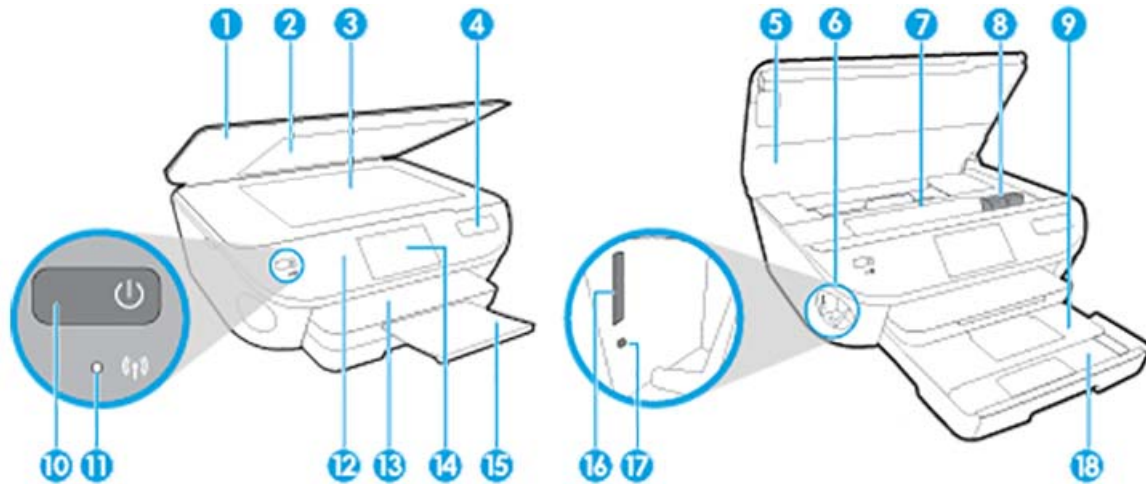
Figur 2-1 HP DeskJet Ink Advantage 5640 All-in-One series set forfra og oppefra
