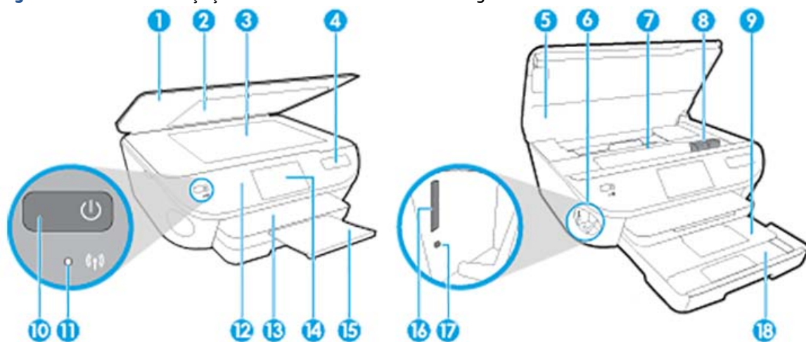
Figura 2-1 Vedere din față și de sus a HP DeskJet Ink Advantage 5640 All-in-One series
