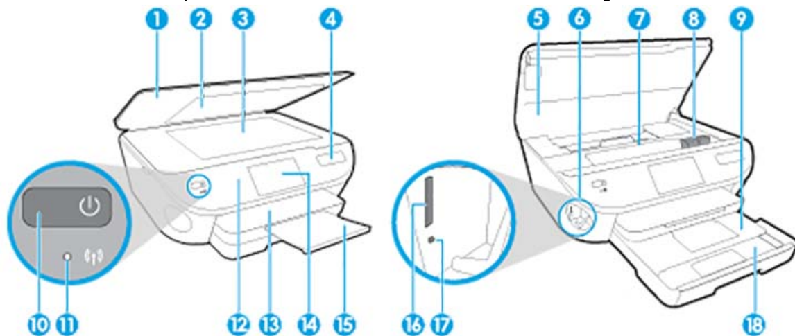
Obrázok 2-1 Pohľad na prednú a hornú časť zariadenia HP DeskJet Ink Advantage 5640 All-in-One series
