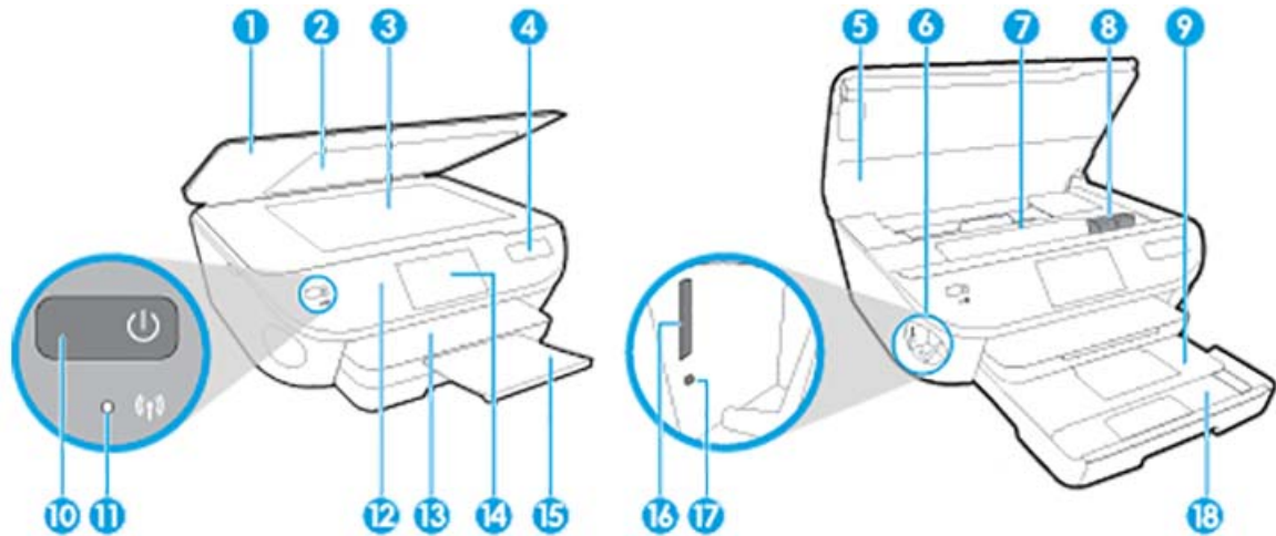
Bild 2-1 HP DeskJet Ink Advantage 5640 All-in-One series sedd framifrån och ovanifrån
