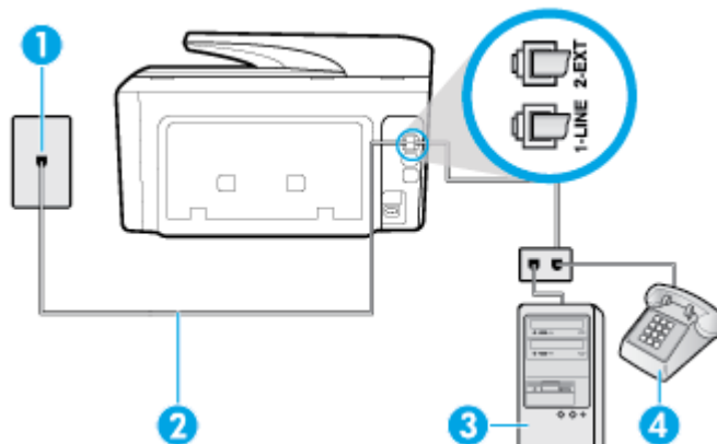
Obrázek 5-16 Zadní pohled na tiskárnu
