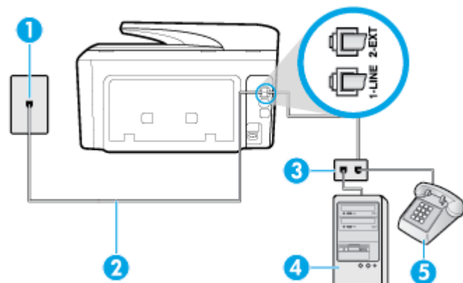
Obrázek 5-9 Zadní pohled na tiskárnu
