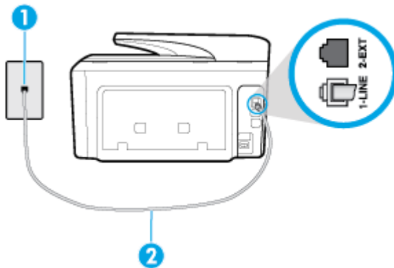
Abbildung 5-3 Rückansicht des Druckers
