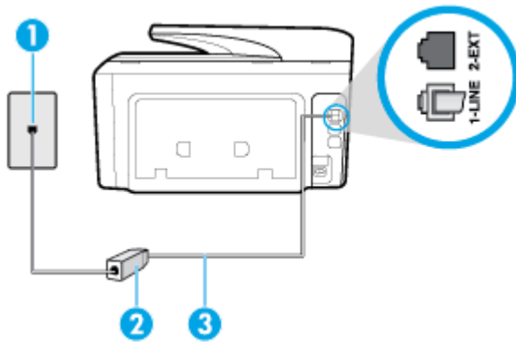
Abbildung 5-2 Rückansicht des Druckers
