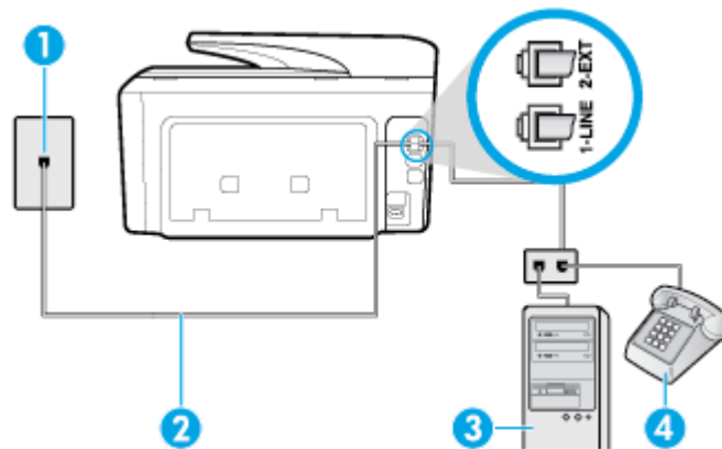
Abbildung 5-16 Rückansicht des Druckers
