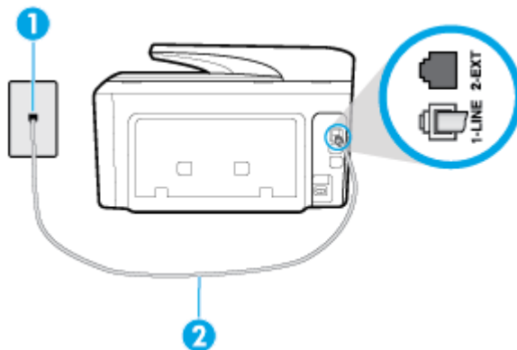
Abbildung 10-1 Rückansicht des Druckers
