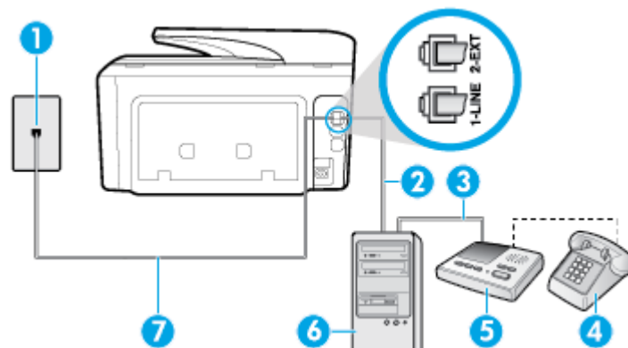
Abbildung 5-13 Rückansicht des Druckers
