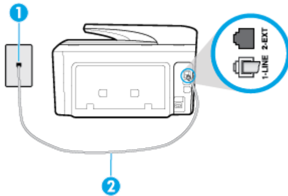
Abbildung 5-5 Rückansicht des Druckers
