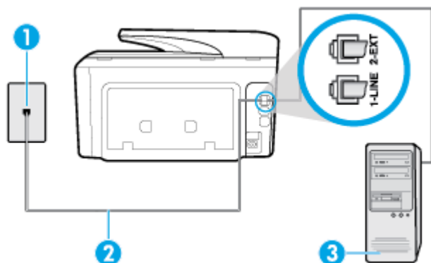
Εικόνα 5-6 Πίσω πλευρά εκτυπωτή
