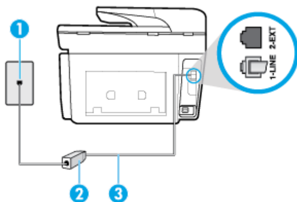
Obrázek 5-2 Zadní pohled na tiskárnu
