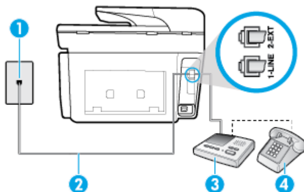
Obrázek 5-11 Zadní pohled na tiskárnu
