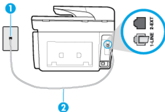
Obrázek 10-1 Zadní pohled na tiskárnu
