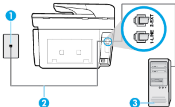
Obrázek 5-6 Zadní pohled na tiskárnu
