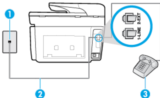
Kuva 5-4 Tulostin takaa
