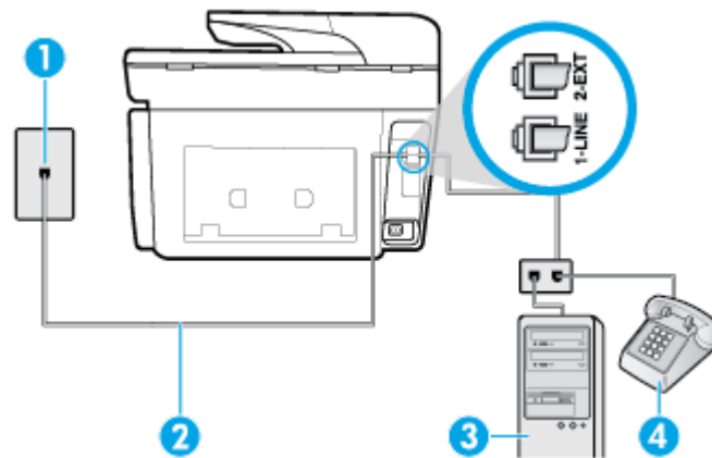
Kuva 5-16 Tulostin takaa
