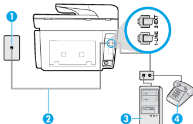
図 5-16 プリンターの背面図
