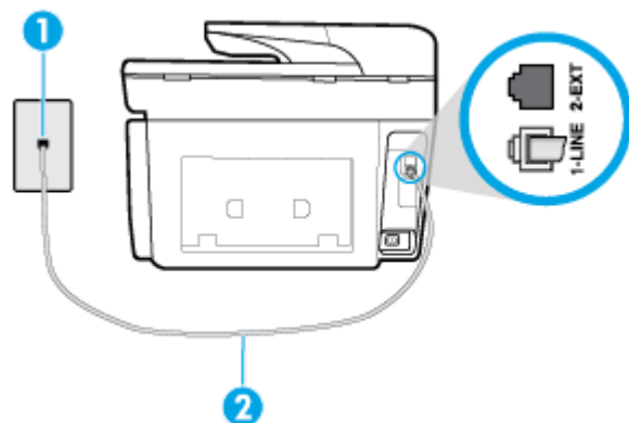
図 5-5 プリンターの背面図
