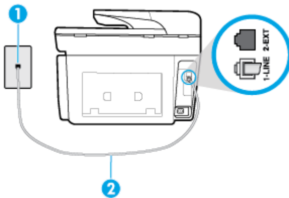
図 5-3 プリンターの背面図
