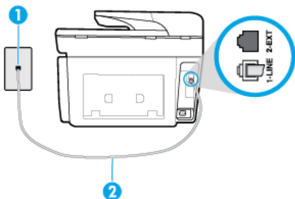
Сурет 10-1 Принтердің артқы көрінісі
