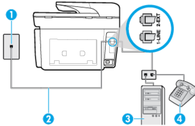
Сурет 5-16 Принтердің артқы көрінісі
