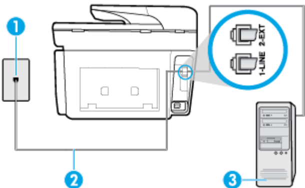
图 5-6 打印机的后视图
