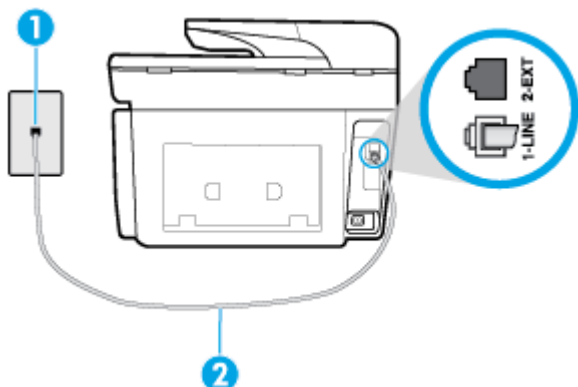
Slika 10-1 Zadnja stran tiskalnika
