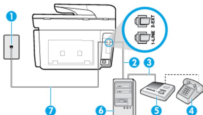
Slika 5-13 Zadnja stran tiskalnika
