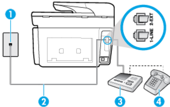
Şekil 5-11 Yazıcının arkadan görünümü
