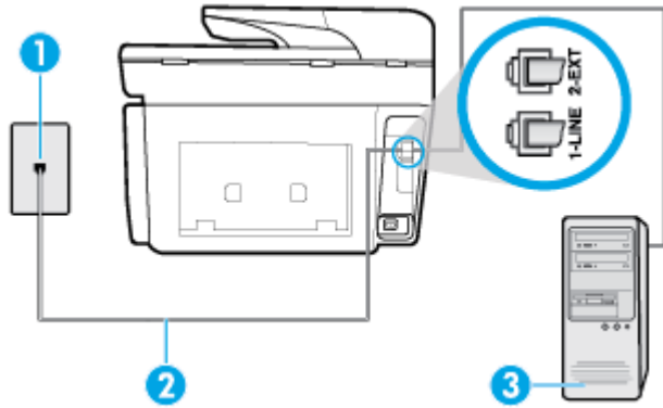
Hình 5-6 Mặt sau của máy in
