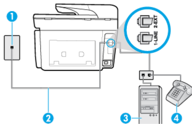
Hình 5-16 Mặt sau của máy in
