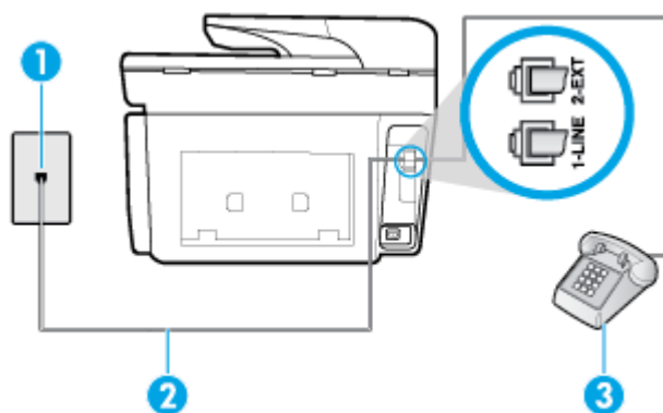
Hình 5-4 Mặt sau của máy in
