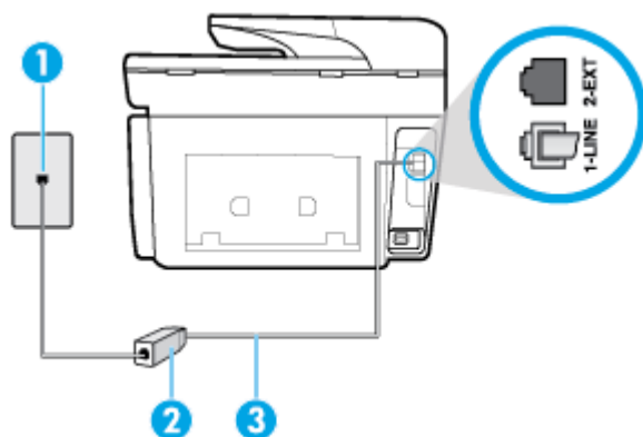
Hình 5-2 Mặt sau của máy in
