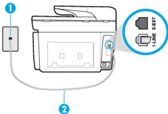
Hình 5-3 Mặt sau của máy in
