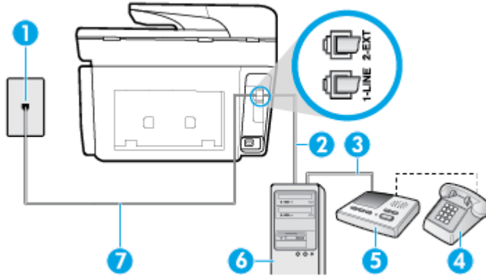
Hình 5-13 Mặt sau của máy in
