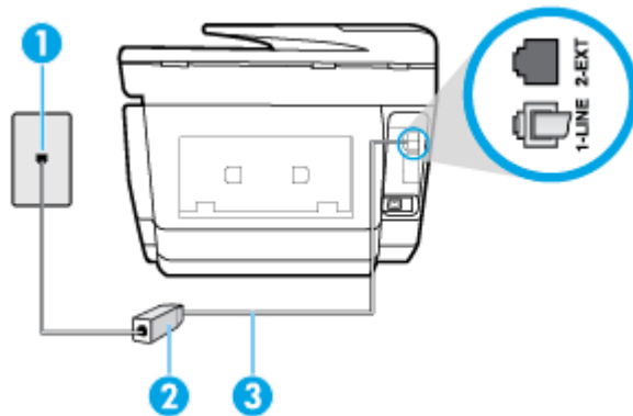
Abbildung 5-2 Rückansicht des Druckers
