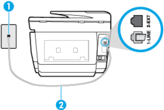
Рисунок 10-1 Вид принтера сзади
