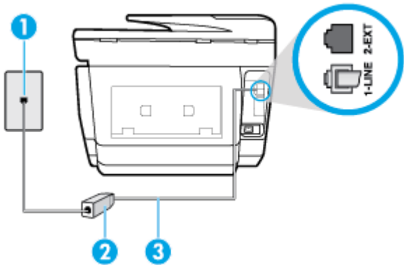
Рисунок 5-2 Вид принтера сзади
