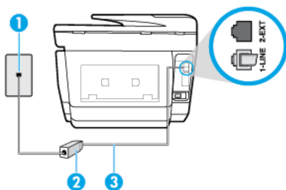
圖示 5-2 印表機的背視圖
