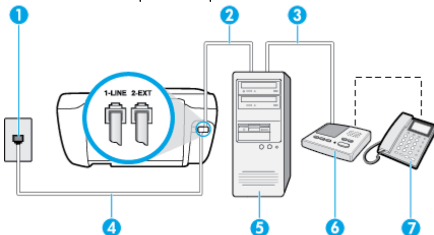
Εικόνα B-13 Πίσω πλευρά εκτυπωτή
