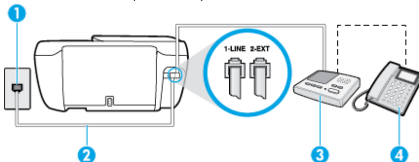
Εικόνα B-11 Πίσω πλευρά εκτυπωτή
