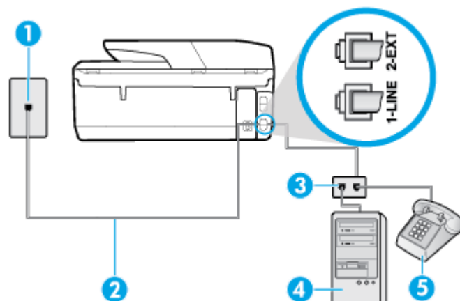
Obrázek 5-9 Zadní pohled na tiskárnu
