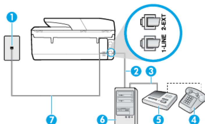
Obrázek 5-13 Zadní pohled na tiskárnu
