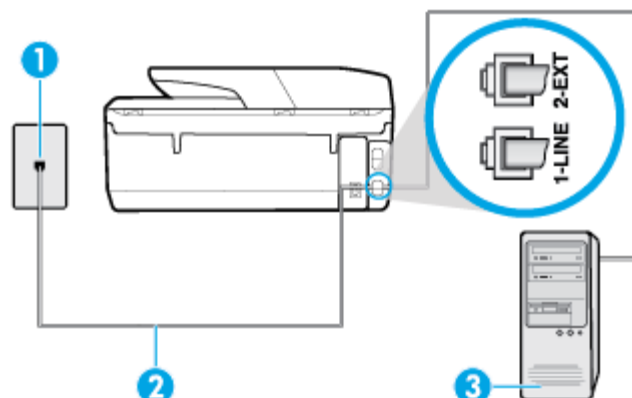
Figura 5-6 Vista posteriore della stampante
