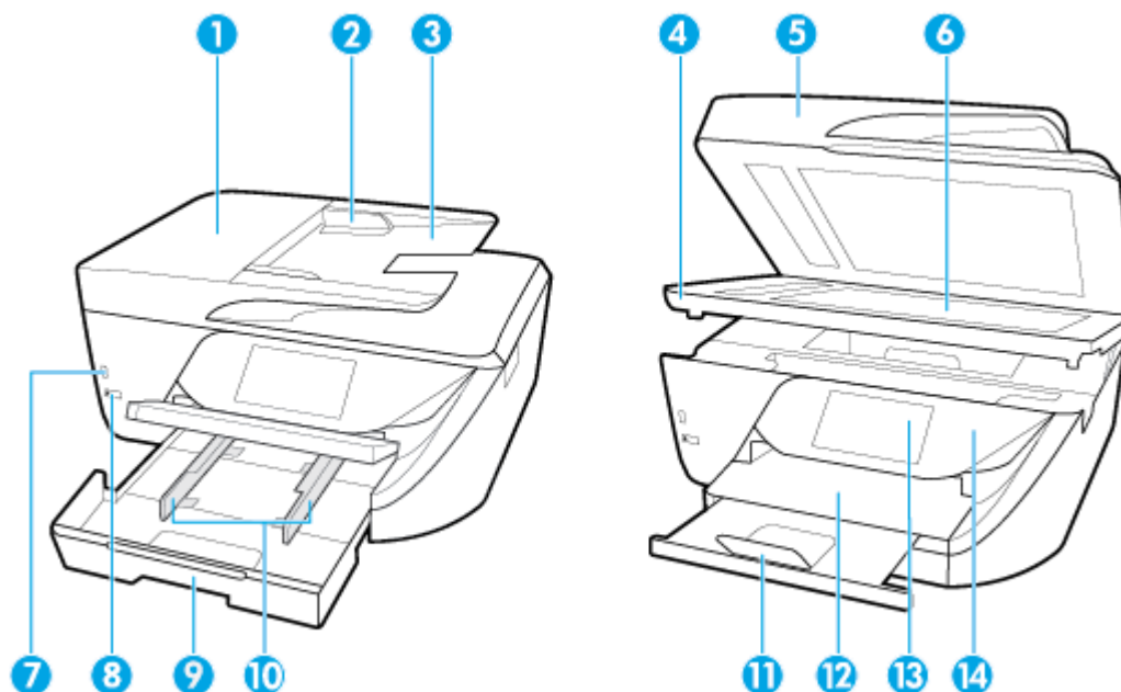
1 文件進紙器
