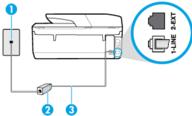
그림 5-2 프린터의 뒷 부분
