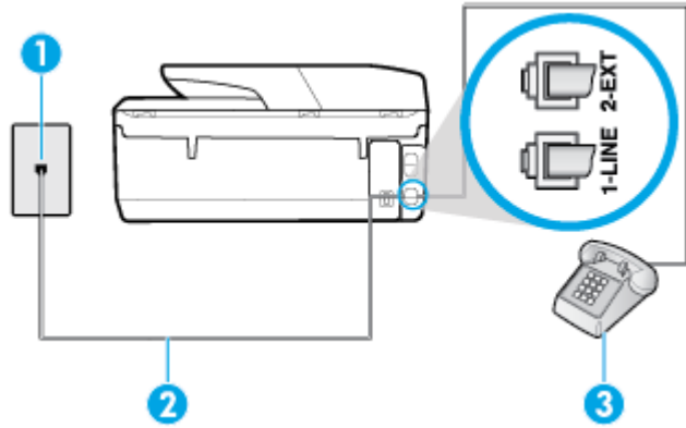
그림 5-4 프린터의 뒷 부분
