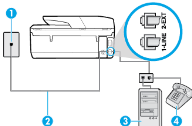
Figur 5-16 Skriveren sett bakfra
