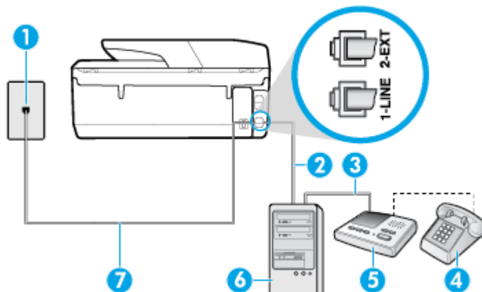
Figur 5-13 Skriveren sett bakfra
