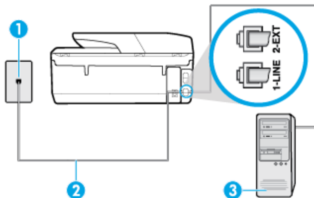
Εικόνα 5-6 Πίσω πλευρά εκτυπωτή
