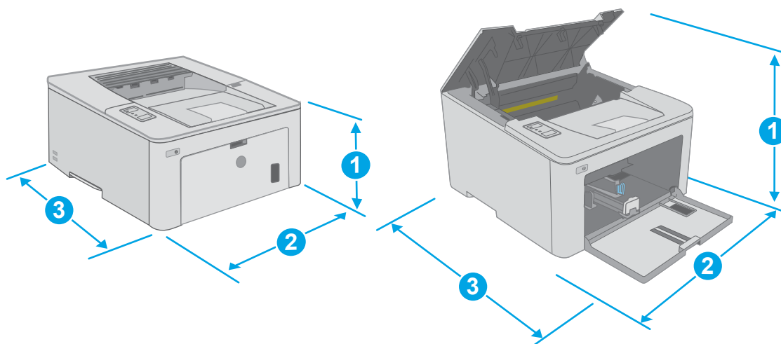
Kuva 1-1 Tulostimen mitat
