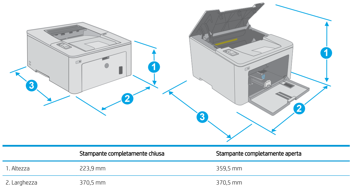
Figura 1-1 Dimensioni per la stampante
