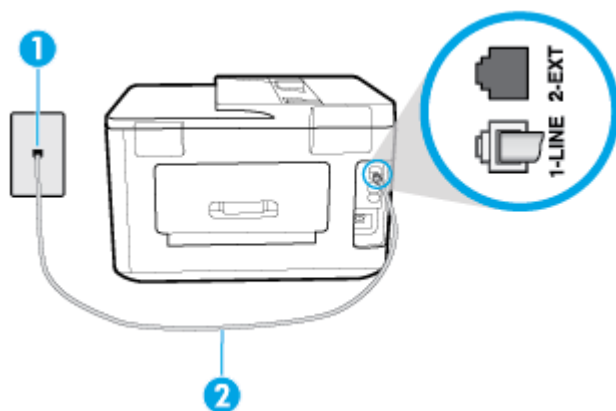
Obrázek 5-1 Zadní pohled na tiskárnu
