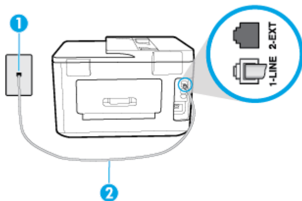
Obrázek 10-1 Zadní pohled na tiskárnu
