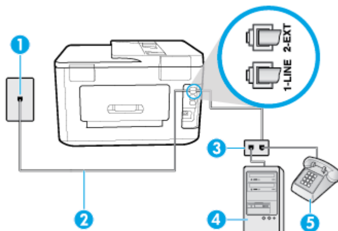
Obrázek 5-9 Zadní pohled na tiskárnu
