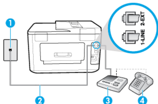
Obrázek 5-11 Zadní pohled na tiskárnu
