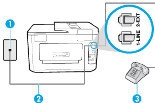
Figura 5-4 Vista posterior de la impresora
