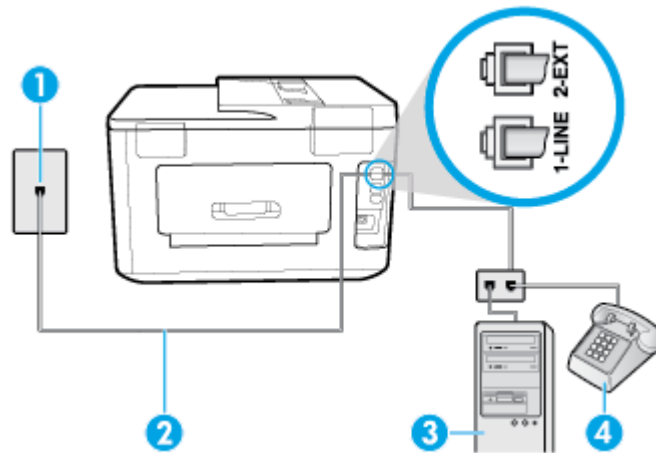
Figura 5-16 Vista posterior de la impresora
