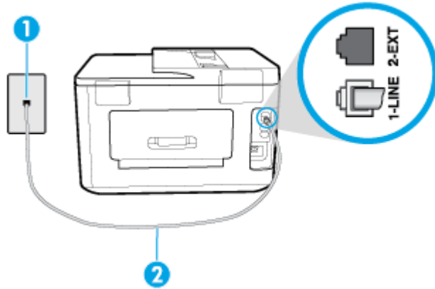
Figura 5-1 Vista posterior de la impresora
