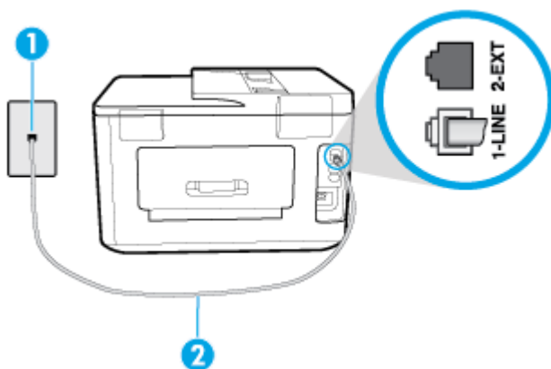
Figura 5-5 Vista posterior de la impresora
