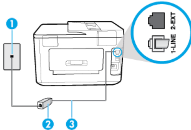
Figura 5-2 Vista posterior de la impresora
