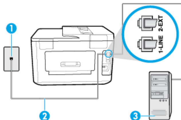
Figura 5-6 Vista posterior de la impresora
