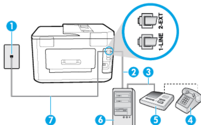
Hình 5-13 Mặt sau của máy in
