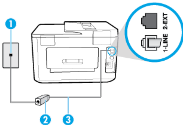
Hình 5-2 Mặt sau của máy in
