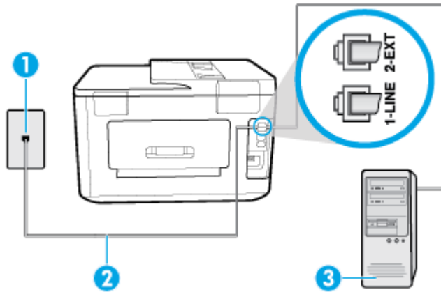
Hình 5-6 Mặt sau của máy in
