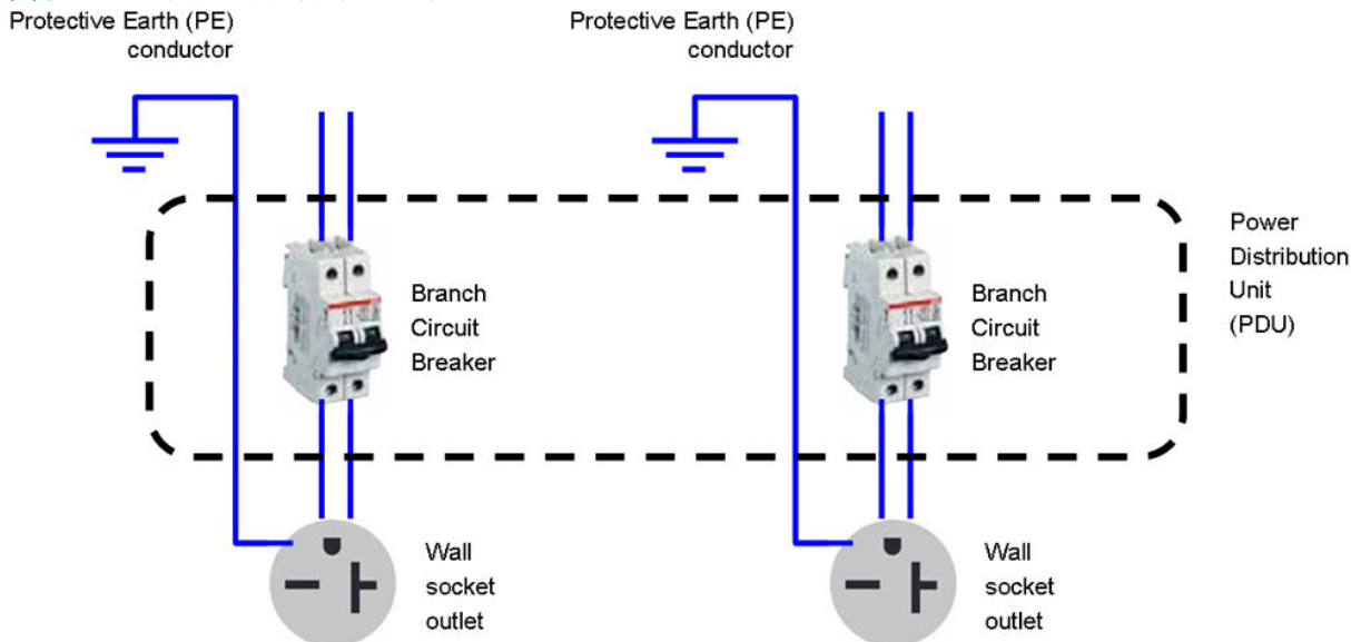
圖示 2-1 電氣設定圖 (僅供參考)
