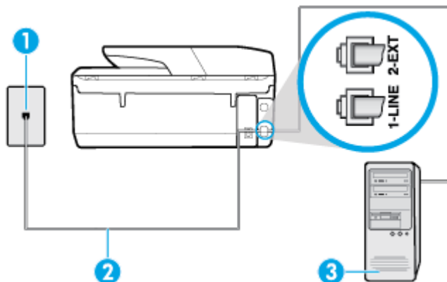
Сурет 5-6 Принтердің артқы көрінісі
