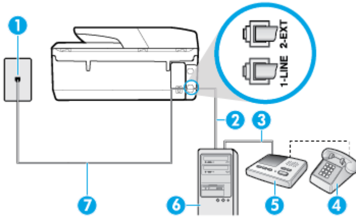
Сурет 5-13 Принтердің артқы көрінісі
