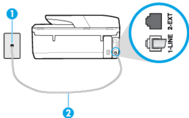
图 5-1 打印机的后视图
