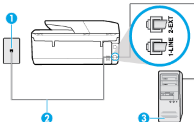
Hình 5-6 Mặt sau của máy in
