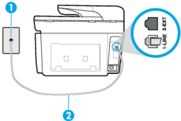
Figure 10-1 Vue arrière de l'imprimante
