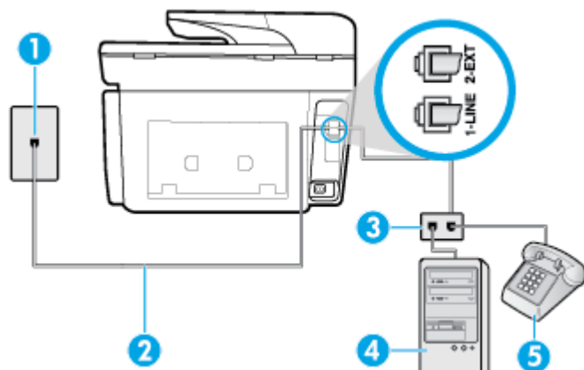
Εικόνα 5-9 Πίσω πλευρά εκτυπωτή
