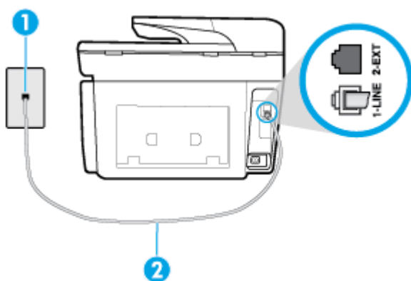
Figur 5-3 Skriveren sett bakfra
