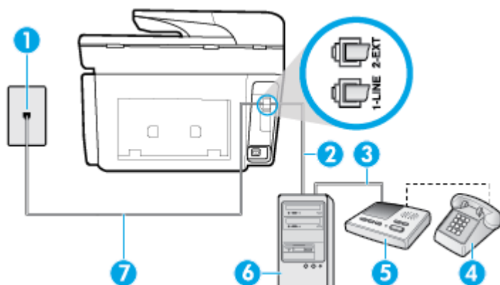
Slika 5-13 Prikaz zadnje strane štampača
