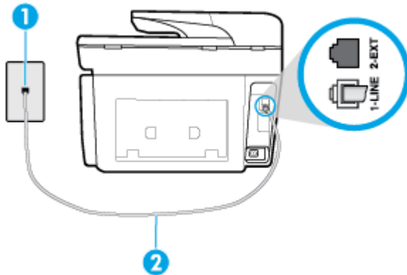
图 5-5 打印机的后视图
