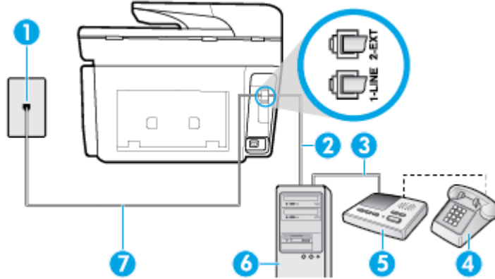
圖示 5-13 印表機的背視圖
