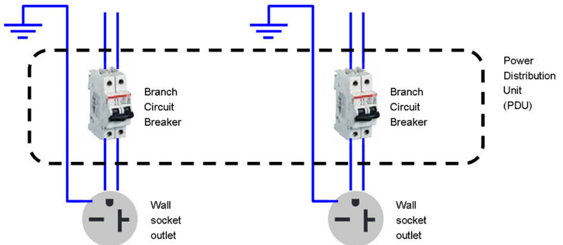
Schéma de configuration électrique (à titre de référence uniquement) Protective Earth (PE) conductor
