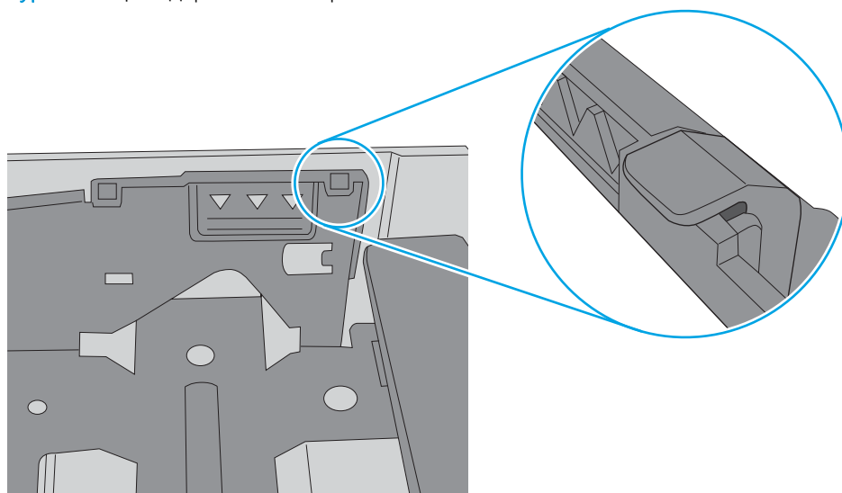
Сурет 9-6 Қағаздар жинағына арналған бекіткіш
