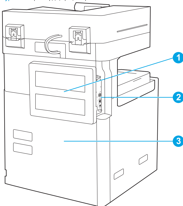
Сурет 1-2 Принтердің артқы көрінісі
